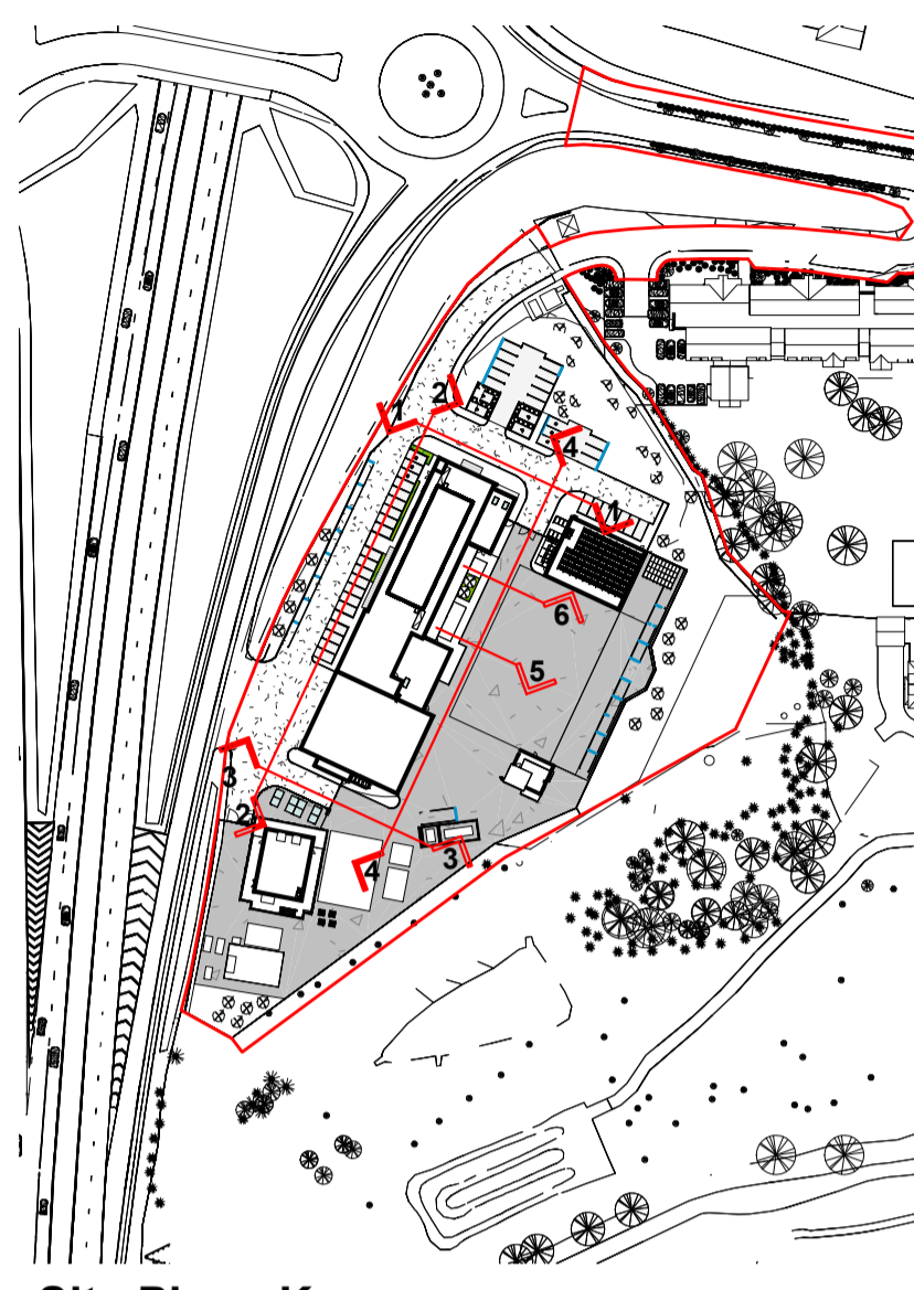
Site Plan - Key 1:2000
